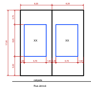
PLANTA ESCALA 1:25
