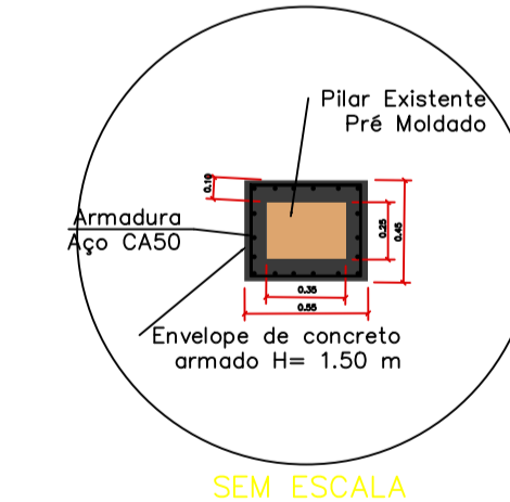
Detalhe A Envolvimento da base de pilar pré moldado
